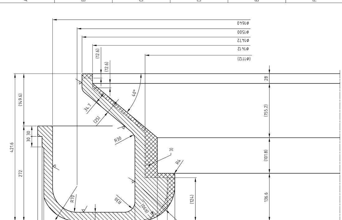
剖视图 A-A 比例 3:10
