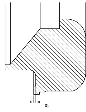
剖视图 D-D
